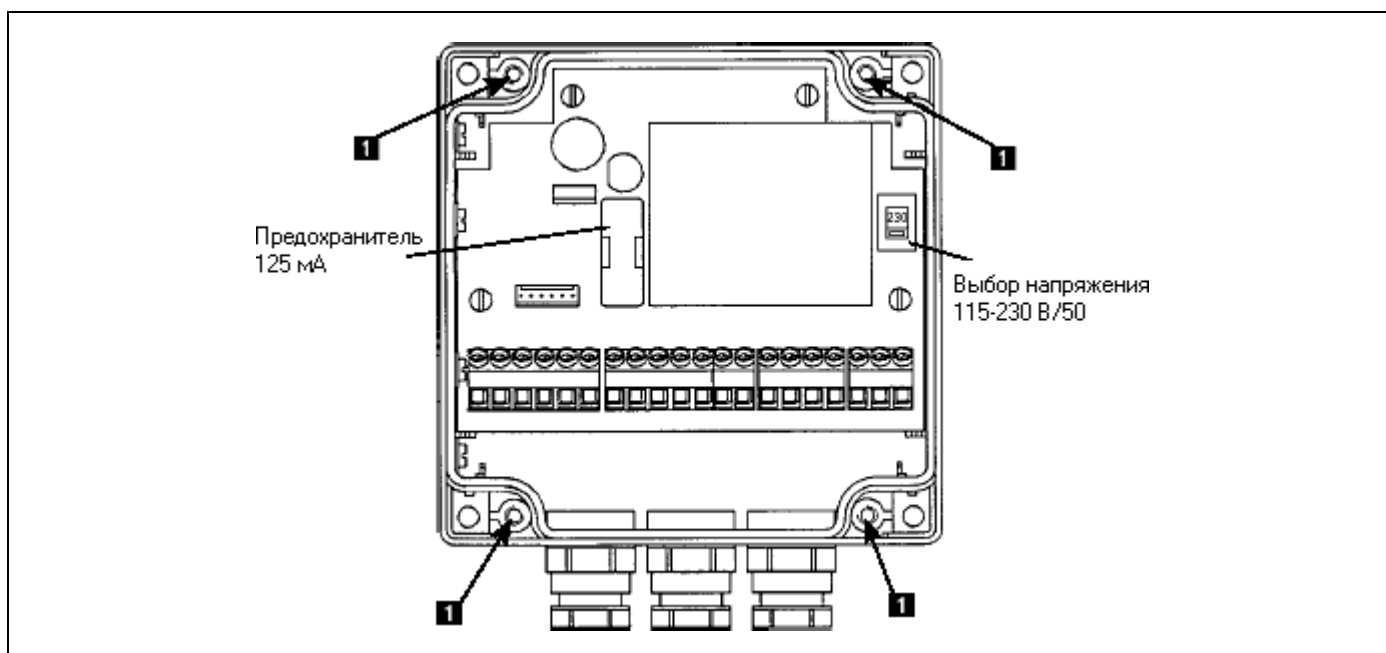
Рис. 3.3 Установка трансмиттера 8225 настенное исполнение
