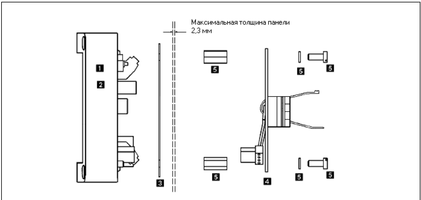
Рис. 5.2 Трансмиситтер 8225 панельное исполнение
